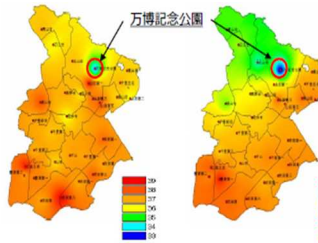
図1 気温分布（8月5日 14時）
