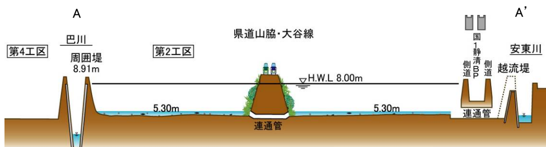
図 4-5 麻機遊水地第2工区横断イメージ図
