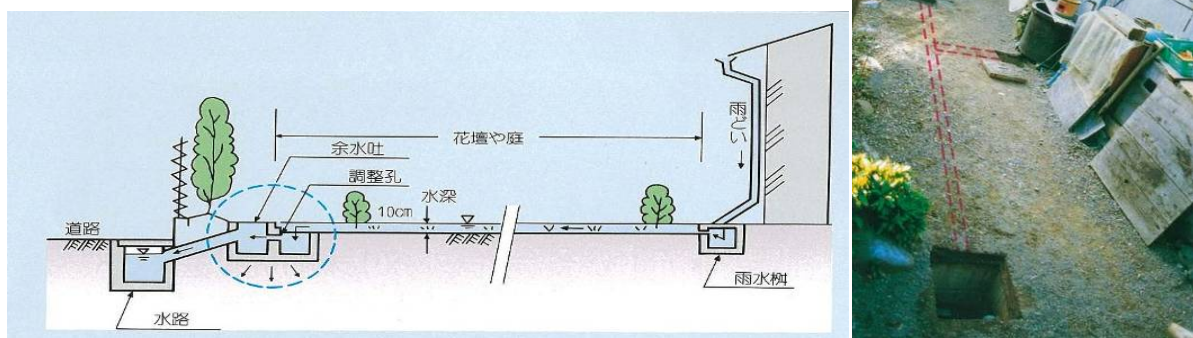
図 2-14 各戸貯留施設の設置状況 -清水区岡町-
