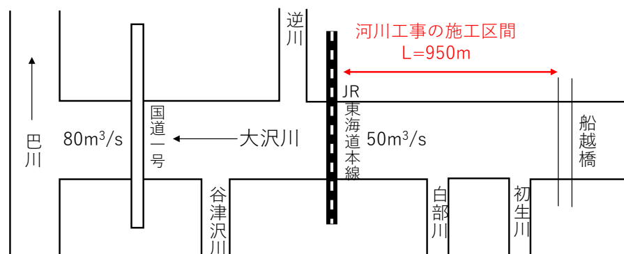
図 4-14 流量配分図
