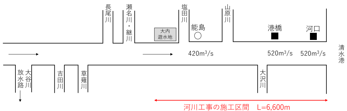
図 4-7 流量配分図
