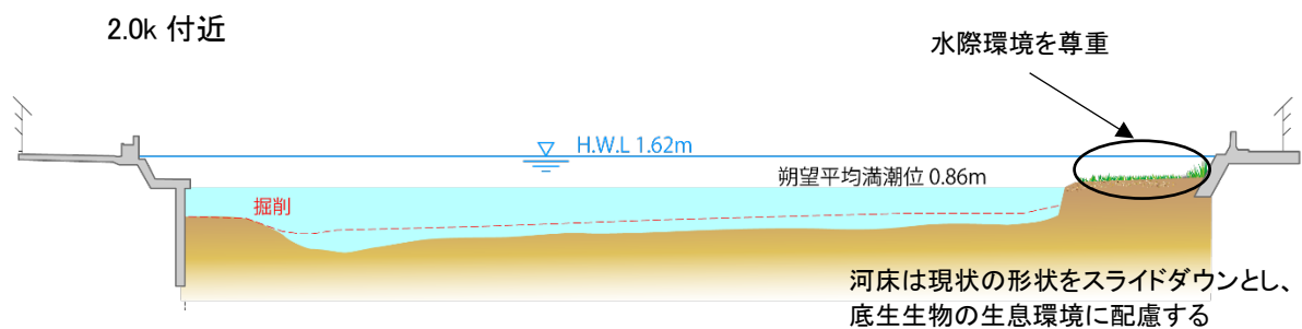
図 4-8 改修横断イメージ図
