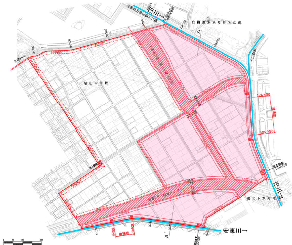
図 4-4 麻機遊水地第2工区平面図
