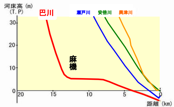
図 1-4 河川縦断図
