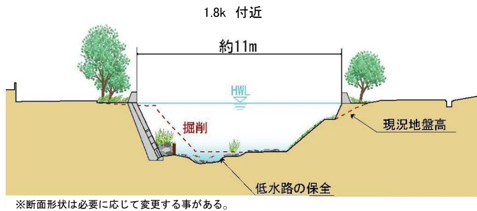
図 4-15 大沢川横断イメージ
