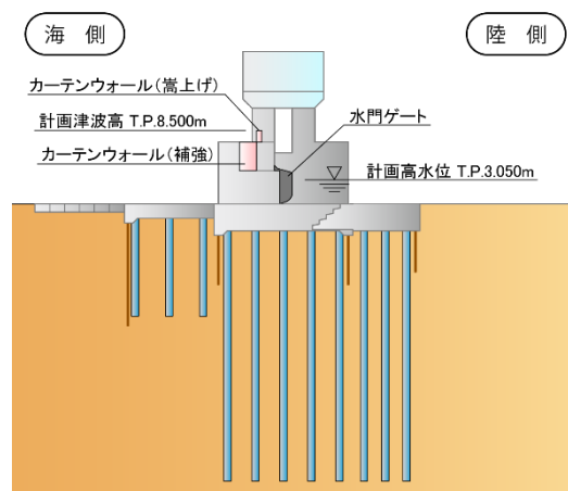
図 4-19 津波対策水門イメージ図
