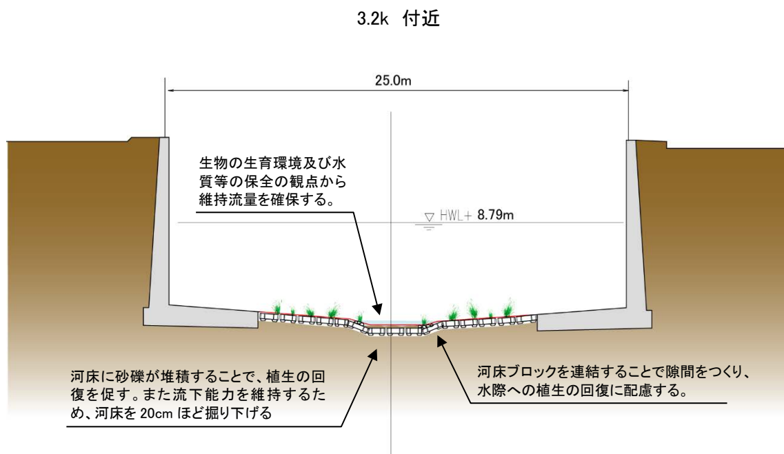
図 4-12 改修横断イメージ図
