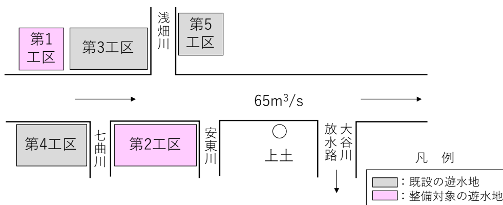
図 4-3 流量配分図
