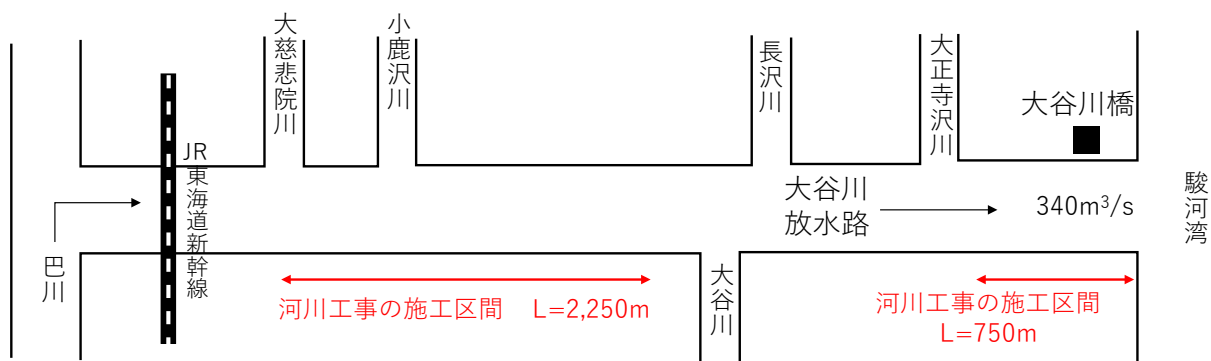
図 4-11 流量配分図
