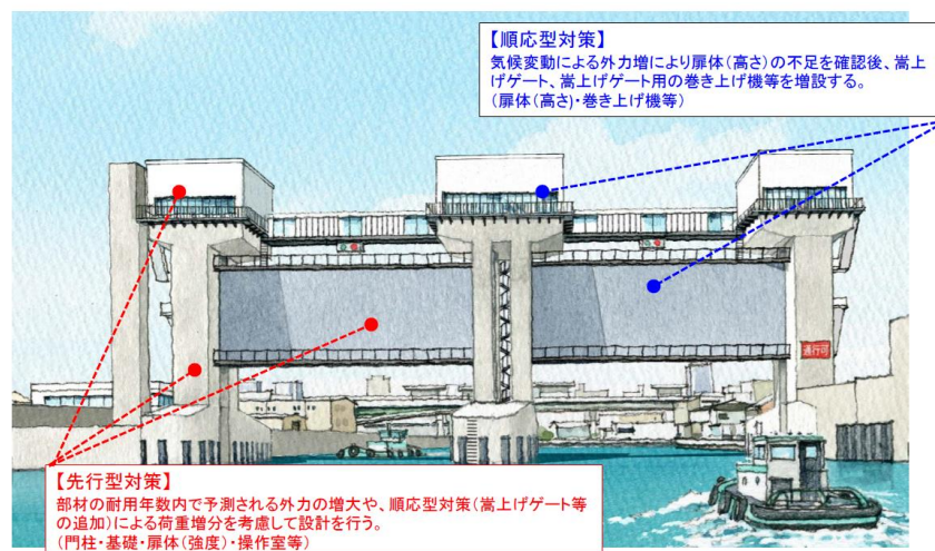
図 49 新木津川水門の設計の考え方(大阪府)
