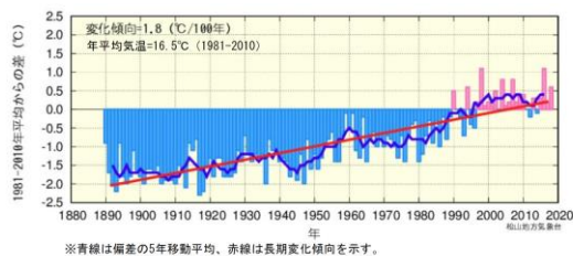
図 13 年平均気温の経年変化 (松山地方気象台)
