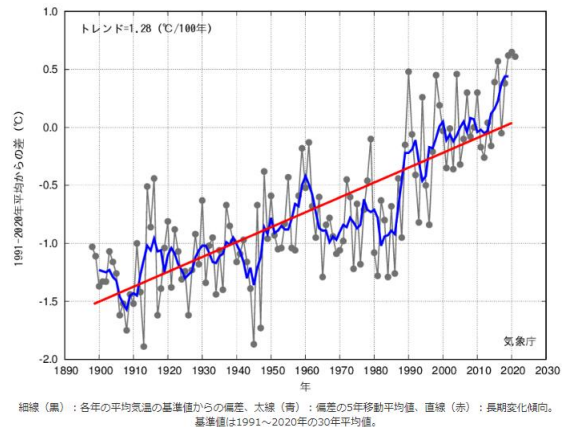
図 16 日本における年平均気温の 1991～2020 年平均からの差
