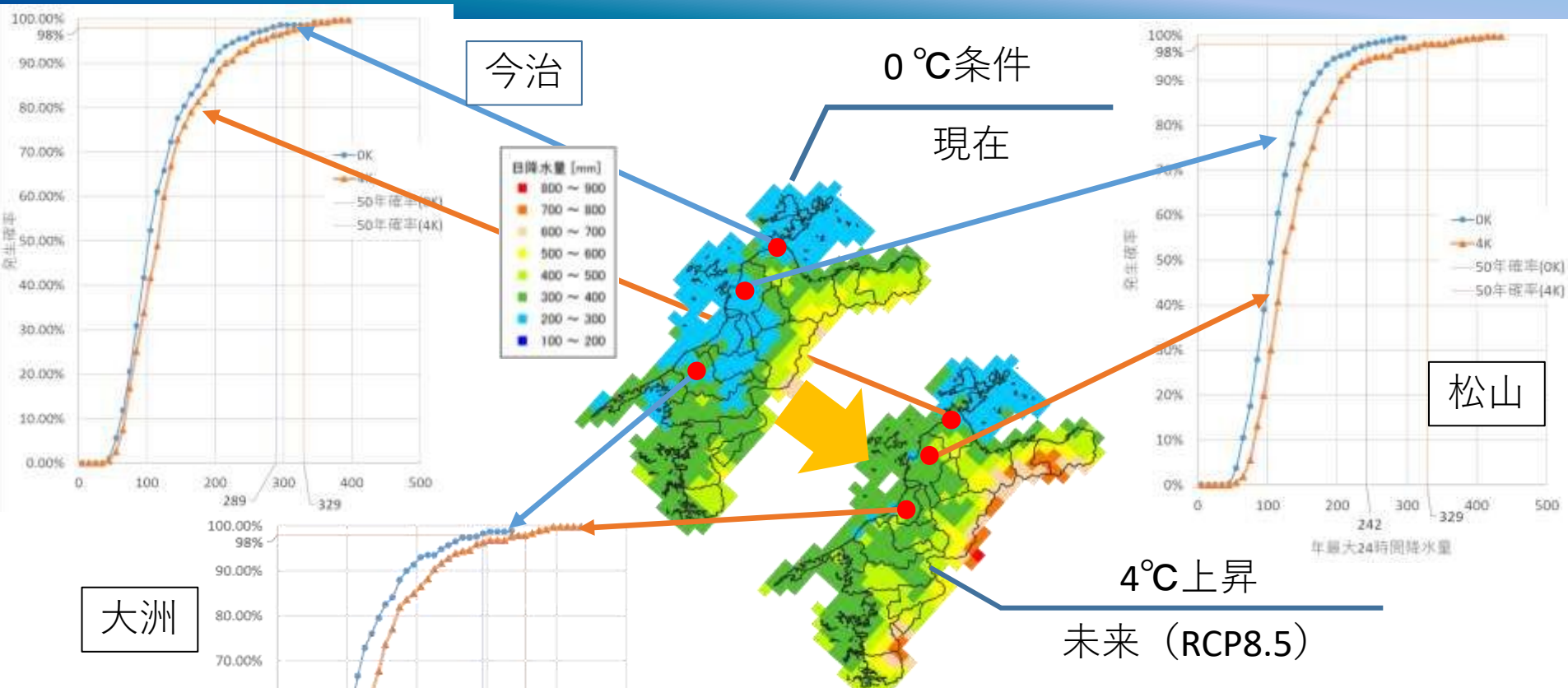
50年に1度の雨量の変化
