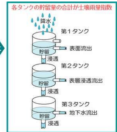
雨が土壌中に貯まっていく様子とタンクモデルとの対応 https://www.jma.go.jp/jma/kishou/now/bosai/dojoshisu.html （気象庁）
