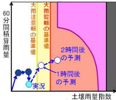
図は「土砂キキクル（大雨警報（土砂災害）の危険度分布）の判定の仕組みから」引用 https://www.jma.go.jp/jma/kishou/now/bosai/doshakeikai.html （気象庁）
