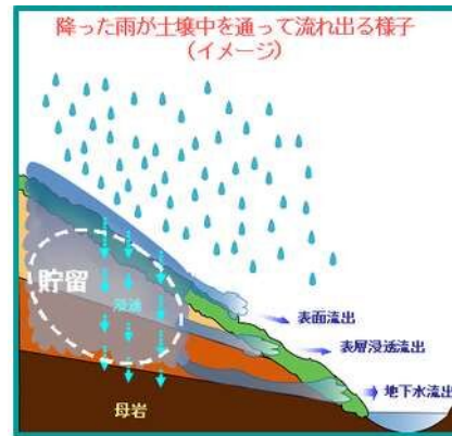
雨が土壌中に貯まっていく様子とタンクモデルとの対応 https://www.jma.go.jp/jma/kishou/now/bosai/dojoshisu.html （気象庁）
