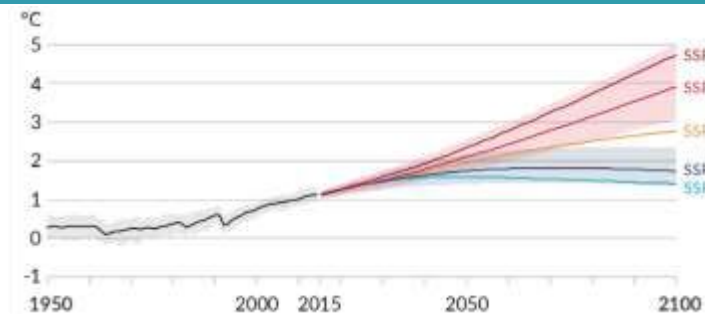
参考：1850-1900年を基準とした世界平均気温の変化 (IPCC WG1 AR6 Figure SPM.8aより)
