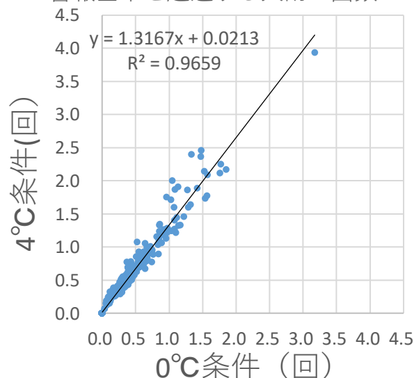
警報基準を超過する大雨の回数
